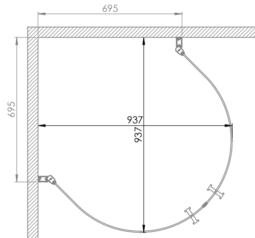
695 x 695 mm symmetrisk montering
