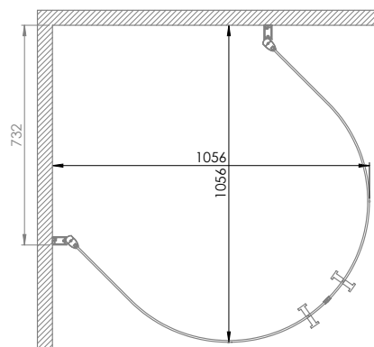
732 x 732 mm symmetrisk montering
